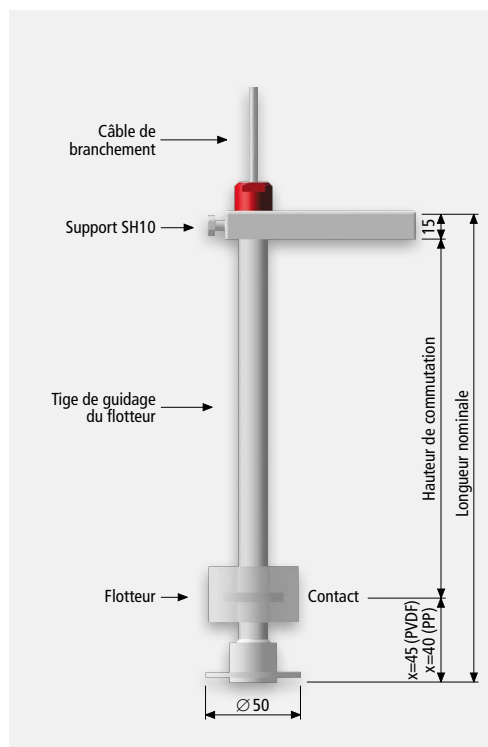
Interrupteur à flotteur avec un point de commutation, en exécution PG
