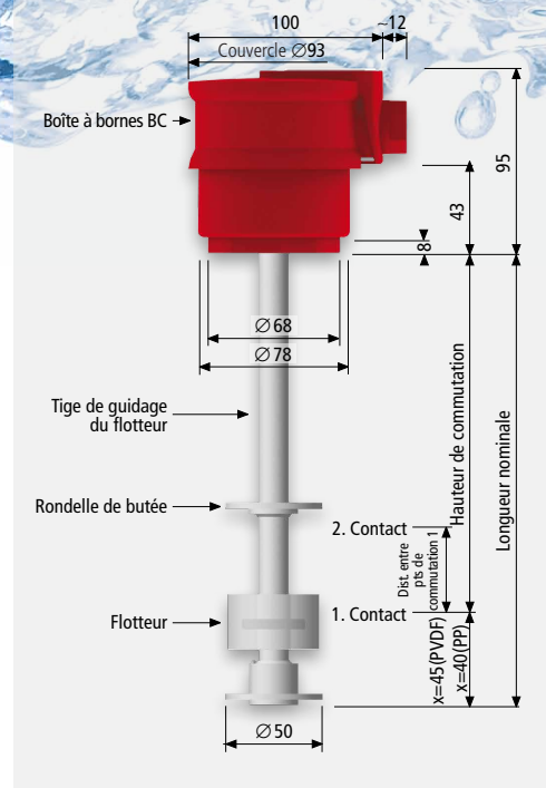
Interrupteur à flotteur avec 2 points de commutation en exécution BC
