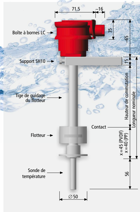
Interrupteur à flotteur avec un point de commutation et sonde de température intégrée, en exécution LC
